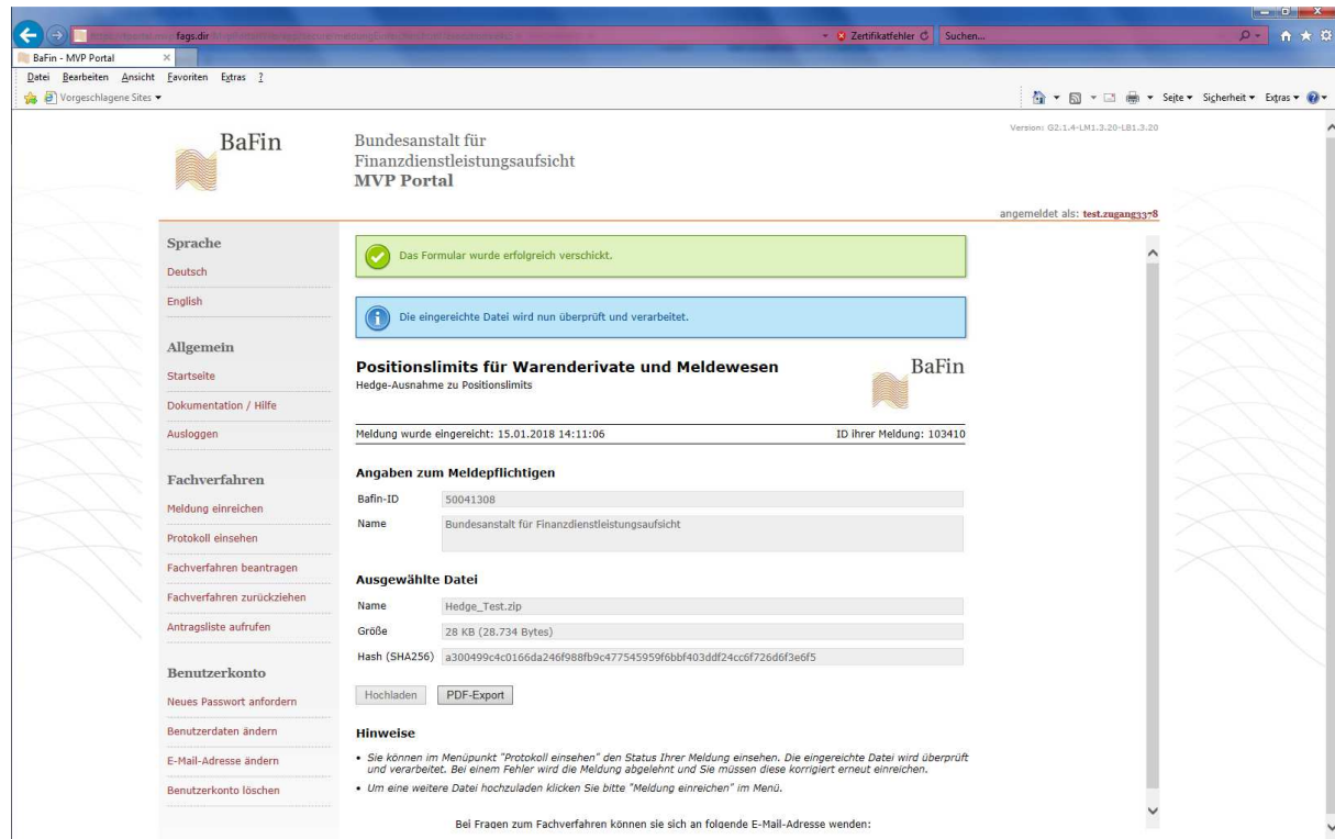
Abbildung 8: Erfolgreicher Upload
