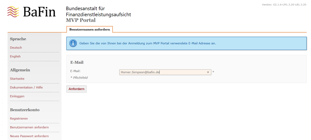
Abbildung 30: Benutzernamen anfordern
